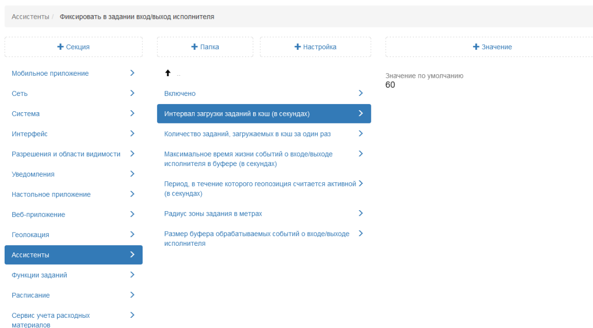
Рис. 2.332: Интервал загрузки заданий в кэш
