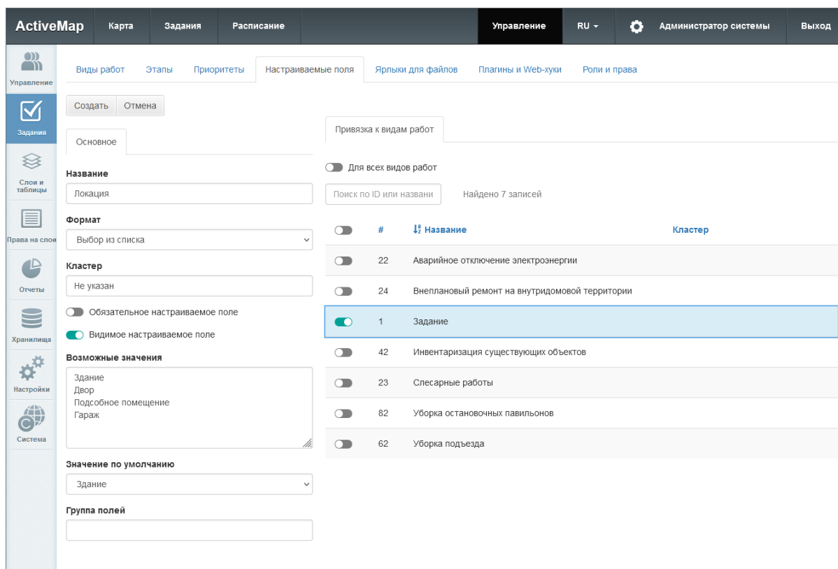
Рис. 2.88: Создание настраиваемого поля, вкладки «Основное» и «Привязка к видам работ»
