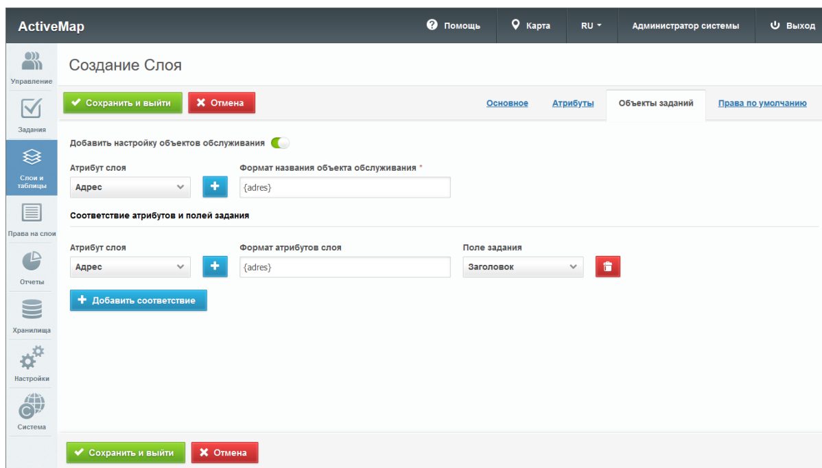
Рис. 2.110: Вкладка «Объекты заданий»
