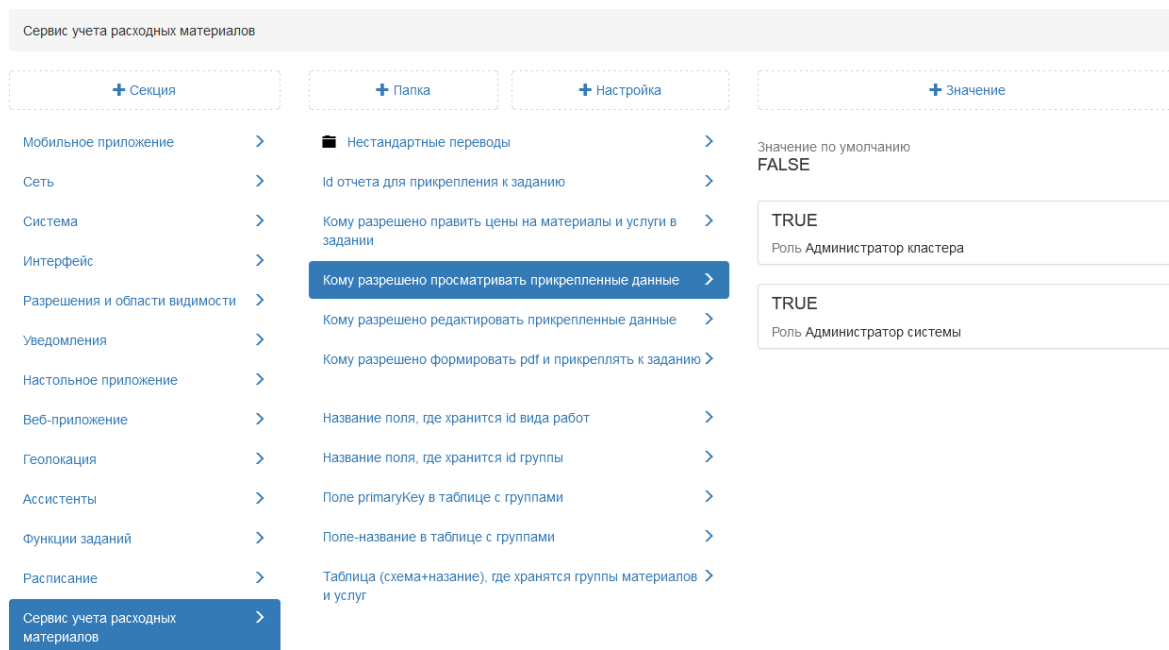
Рис. 2.352: Предоставление доступа для просмотра счет-фактуры
