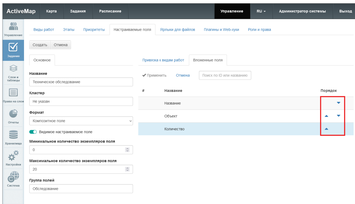
Рис. 2.91: Сортировка вложенных полей
