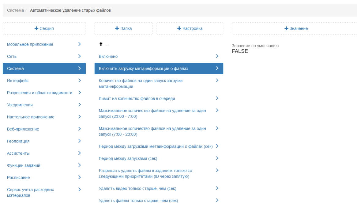
Рис. 2.199: Включить загрузку метаданных о файлах
