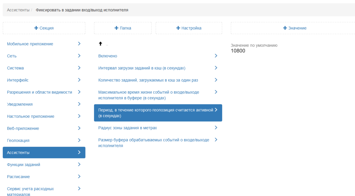
Рис. 2.335: Период, в течение которого геопозиция считается активной
