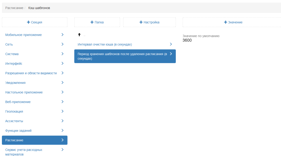
Рис. 2.345: Период хранения шаблонов после удаления расписания (в секундах)
