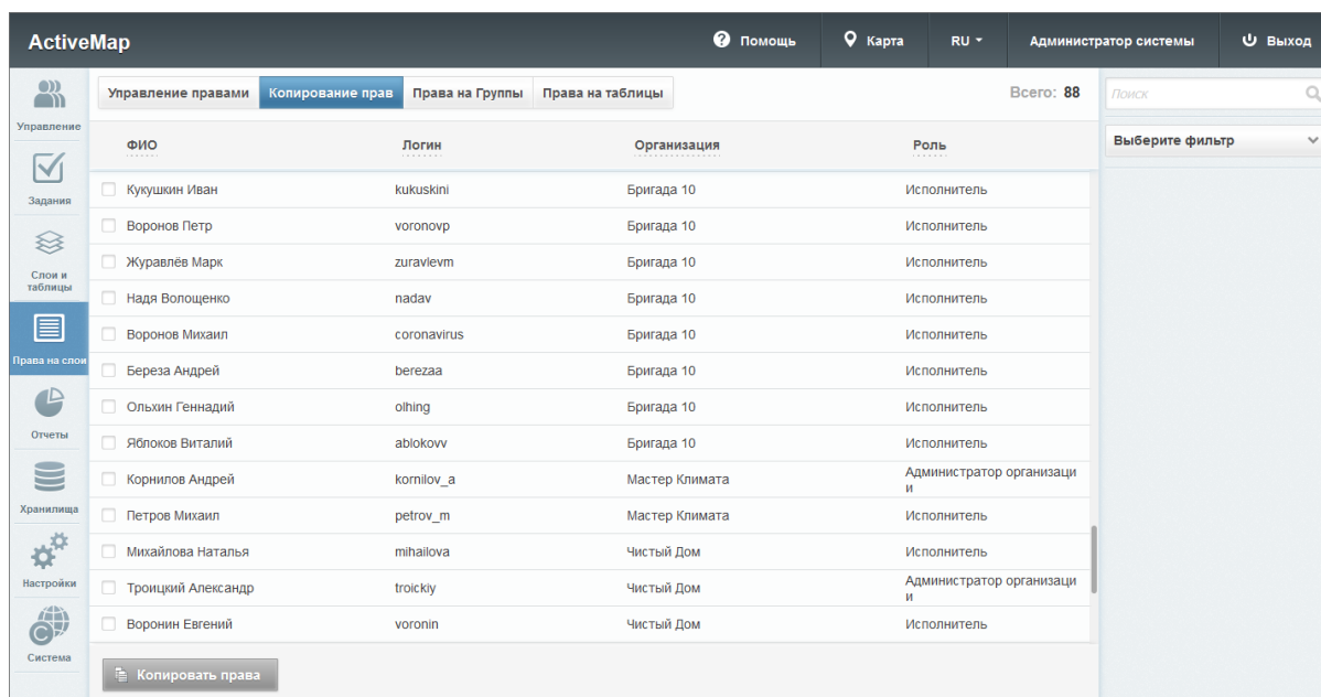
Рис. 2.140: Вкладка «Копирование прав»
