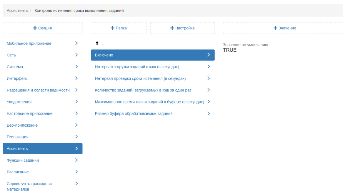
Рис. 2.323: Контроль истечения срока выполнения заданий
