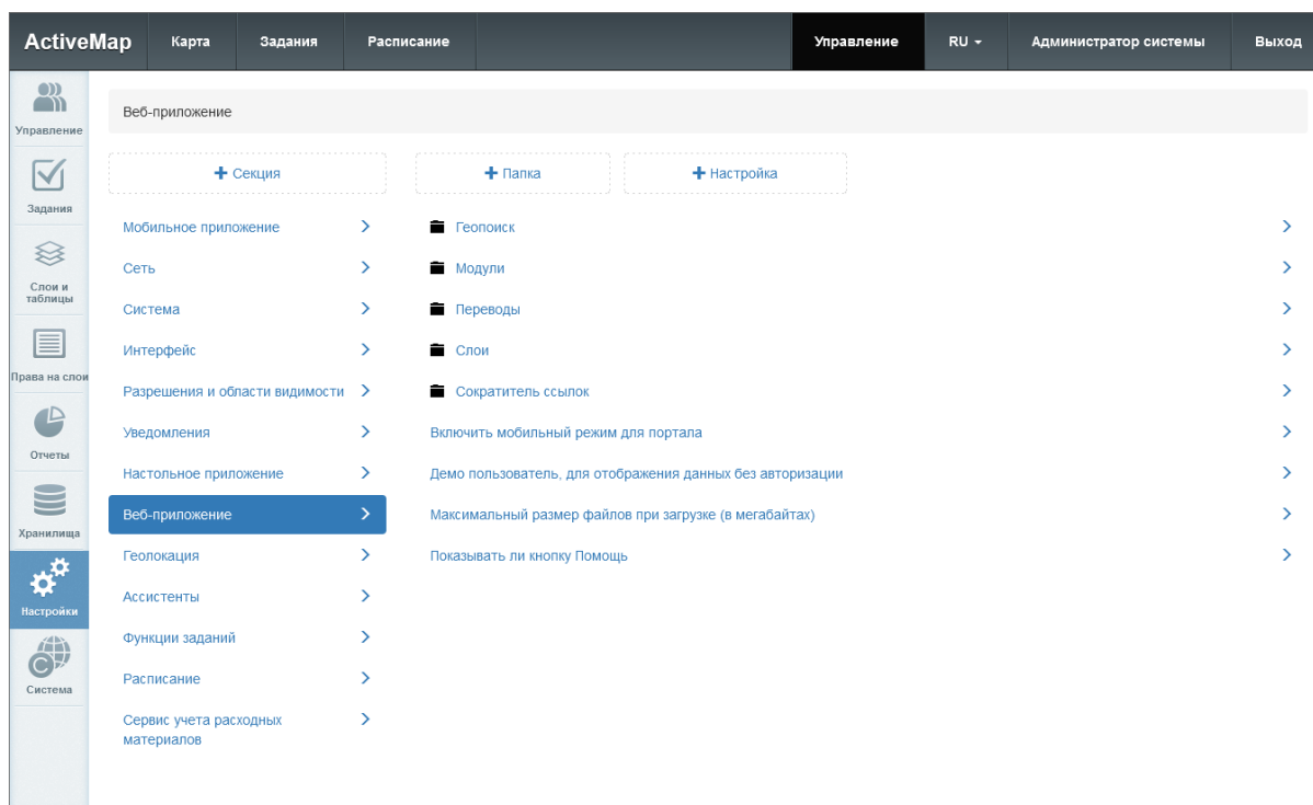
Рис. 2.152: Структура блока «Настройки»
