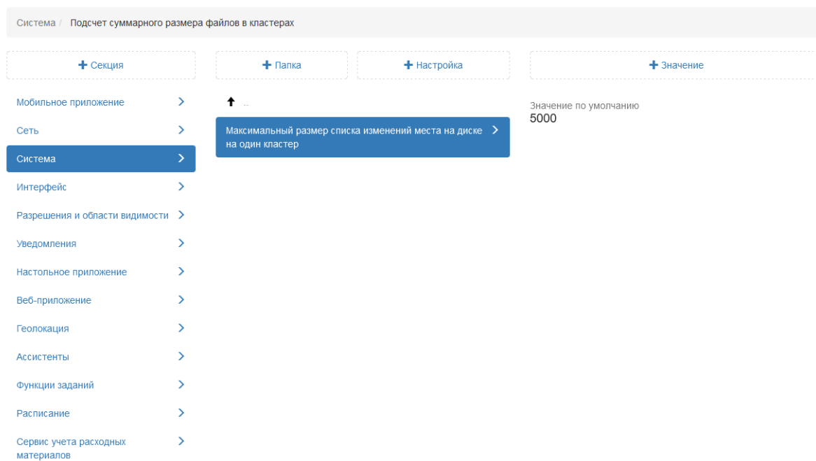
Рис. 2.217: Настройка максимального размера списка изменений места на диске на один кластер
