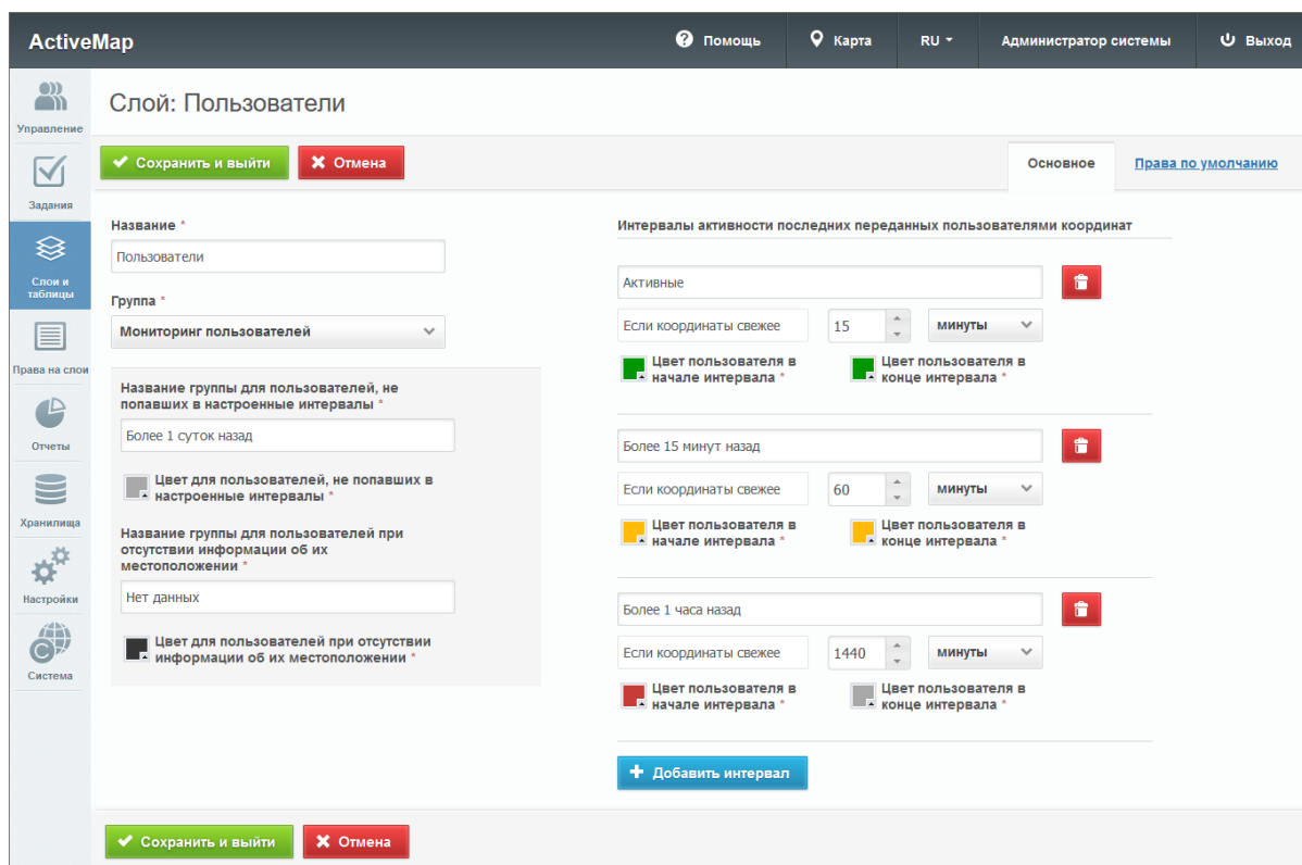
Рис. 2.128: Редактирование системного слоя «Пользователи», вкладка «Основное»
