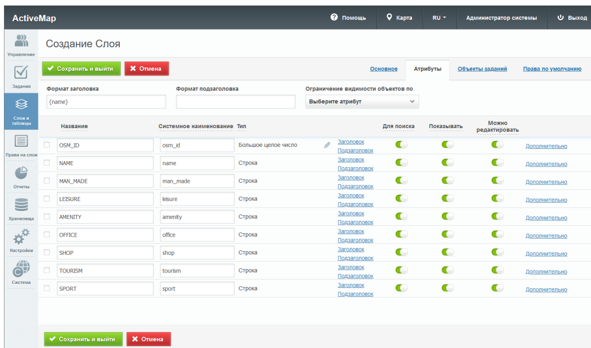
Рис. 2.114: Атрибуты загружаемого слоя
