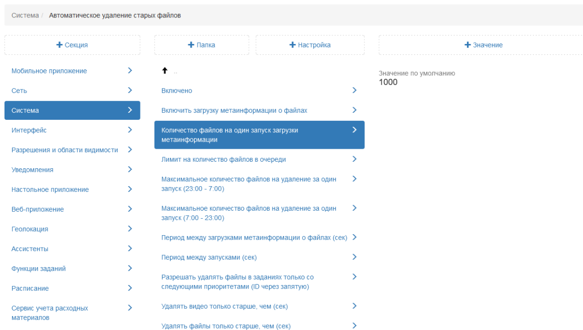
Рис. 2.200: Количество файлов на один запуск загрузки метаинформации
