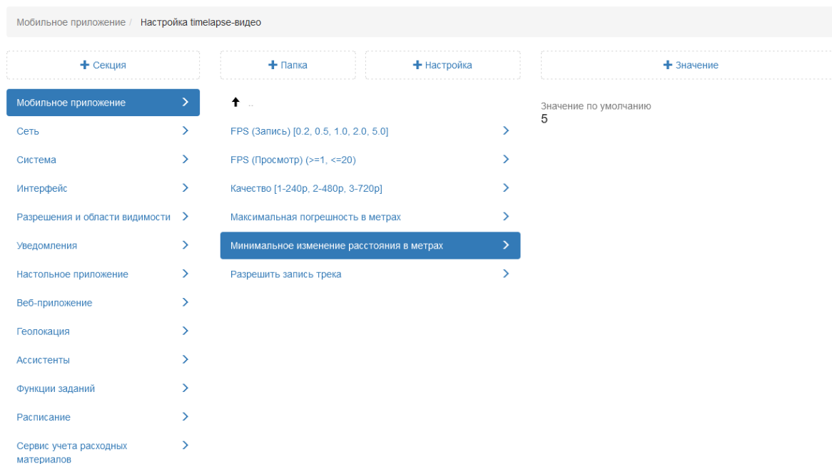
Рис. 2.182: Максимальная погрешность в метрах
