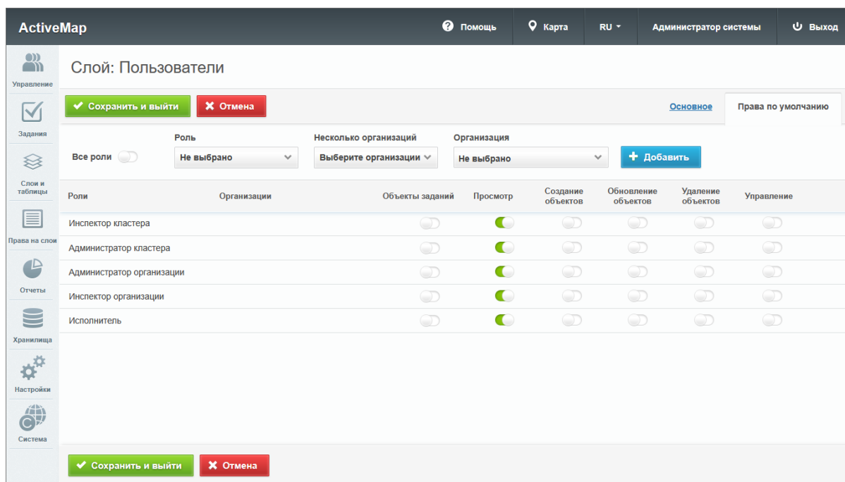
Рис. 2.129: Редактирование системного слоя «Пользователи», вкладка «Права по умолчанию»
