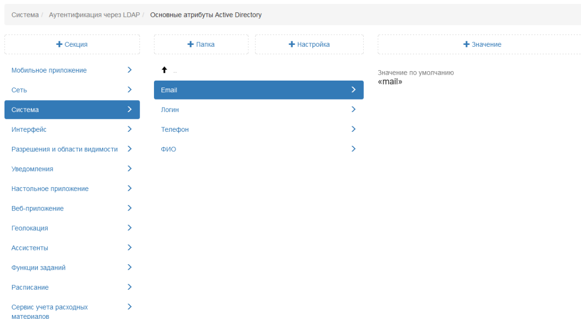
Рис. 2.212: Основные атрибуты Active Directory
