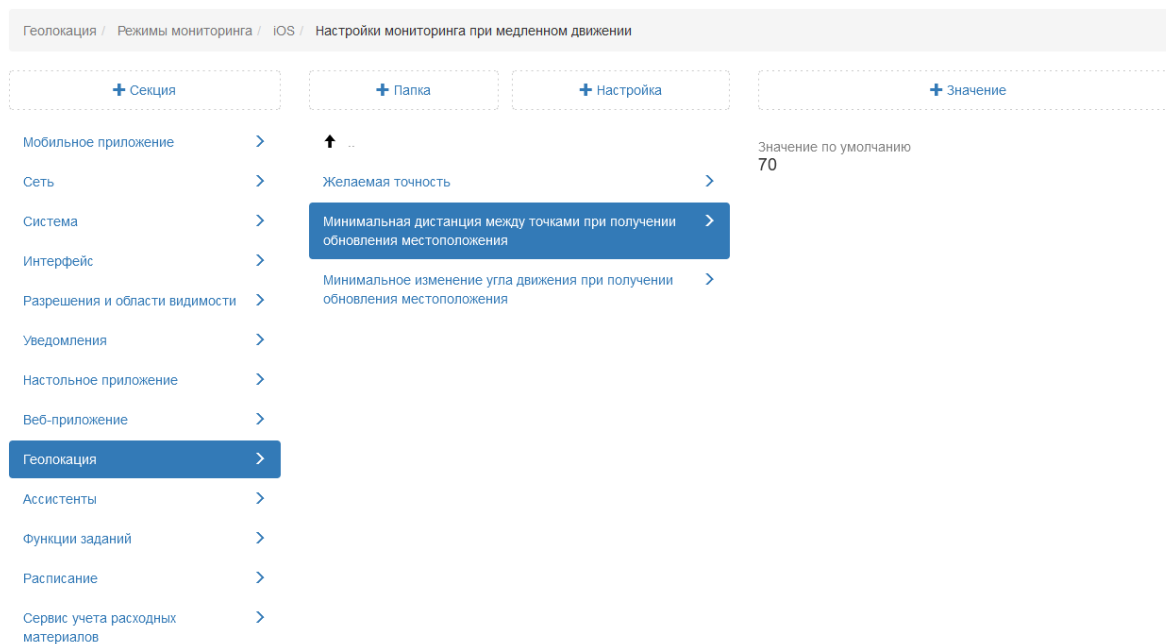
Рис. 2.302: Минимальная дистанция между точками при получении обновления местоположения
