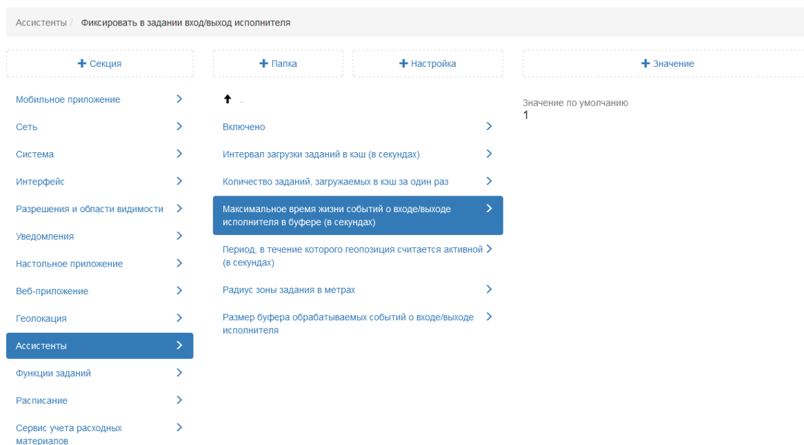
Рис. 2.334: Максимальное время жизни событий о входе/выходе исполнителя в буфере (в секундах)
