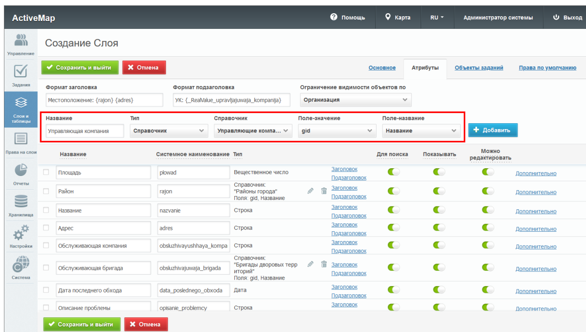
Рис. 2.107: Прикрепление справочника к полю слоя
