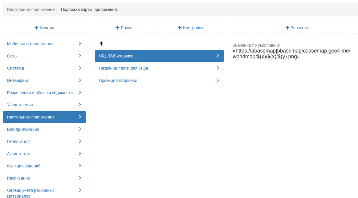
Рис. 2.250: Подложка карты приложения
