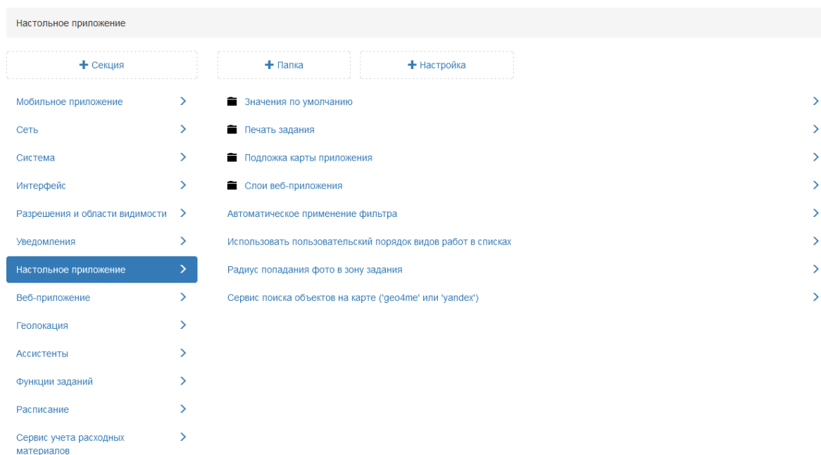
Рис. 2.244: Секция «Настольное приложение»
